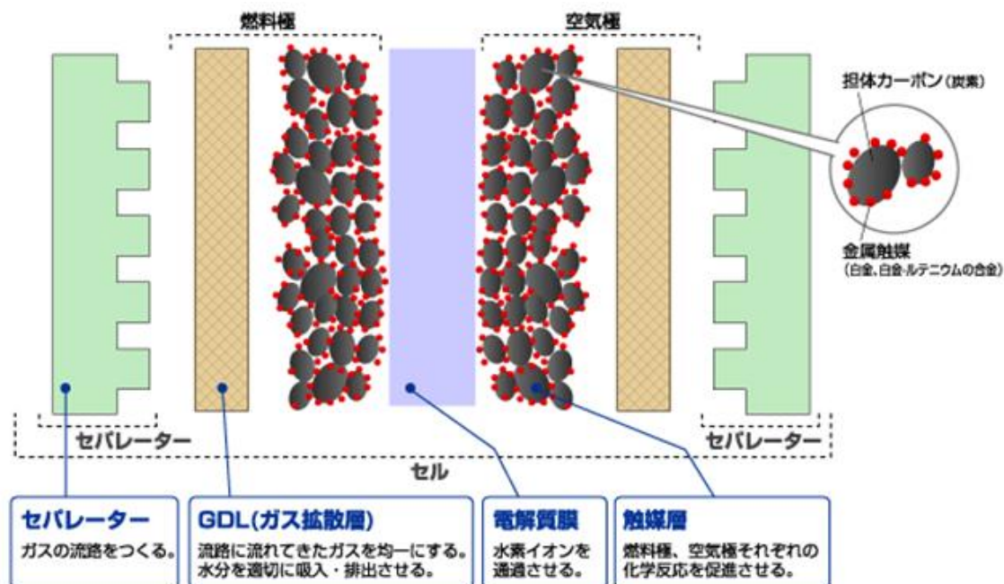
図 3 燃料電池の内部構造
