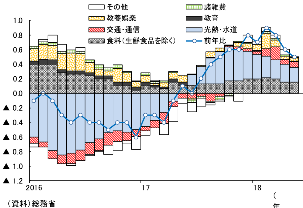
(図表2)東京都区部消費者物価指数(生鮮食品を除く総合)
